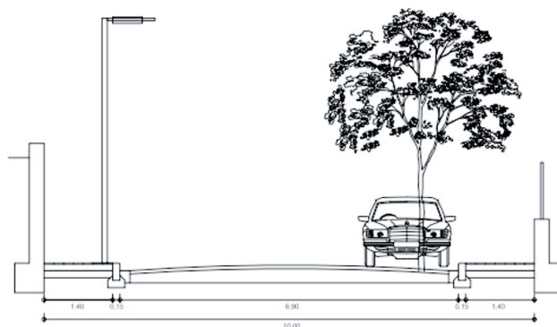
Secció del carrer segons projecte
